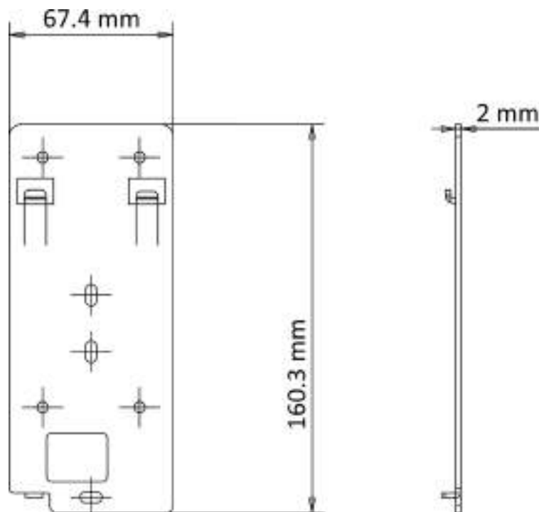
Рисунок 3-1. Монтажная плата
