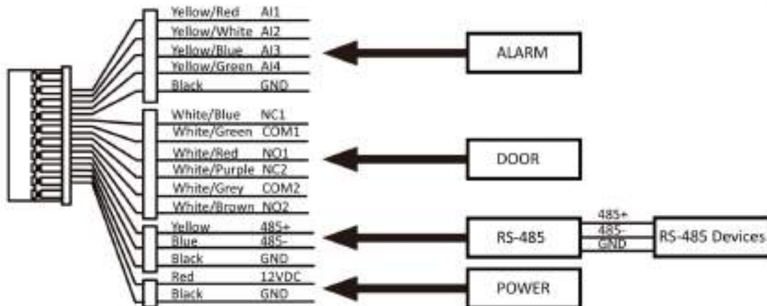
Рисунок 2-1. Описание разъемов
